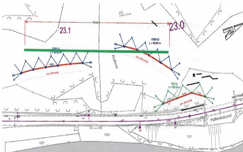
Lage der projektierten Steinschlagverbauungen (rote Linien) mit Verankerungen (blau). Die geoelektrische Messlinie (grüne Gerade) soll etwas oberhalb der Verbauungen ausgeführt werden. (Fig. 1.1 des Berichts zur geoelektrischen Untersuchung, 31. Mai 2024)
