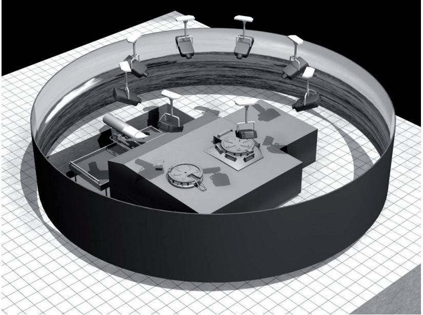
Nouvelle installation électronique d'instruction au tir Leopard
