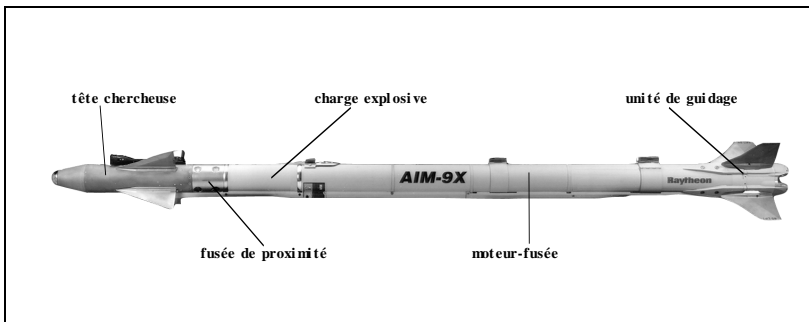
Le missile Sidewinder AIM-9X comporte cinq groupes d'assemblage principaux.
