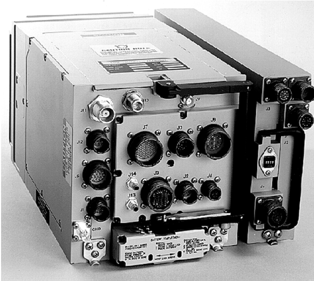
Terminal MIDS pour le transfert de données résistant au brouillage.
