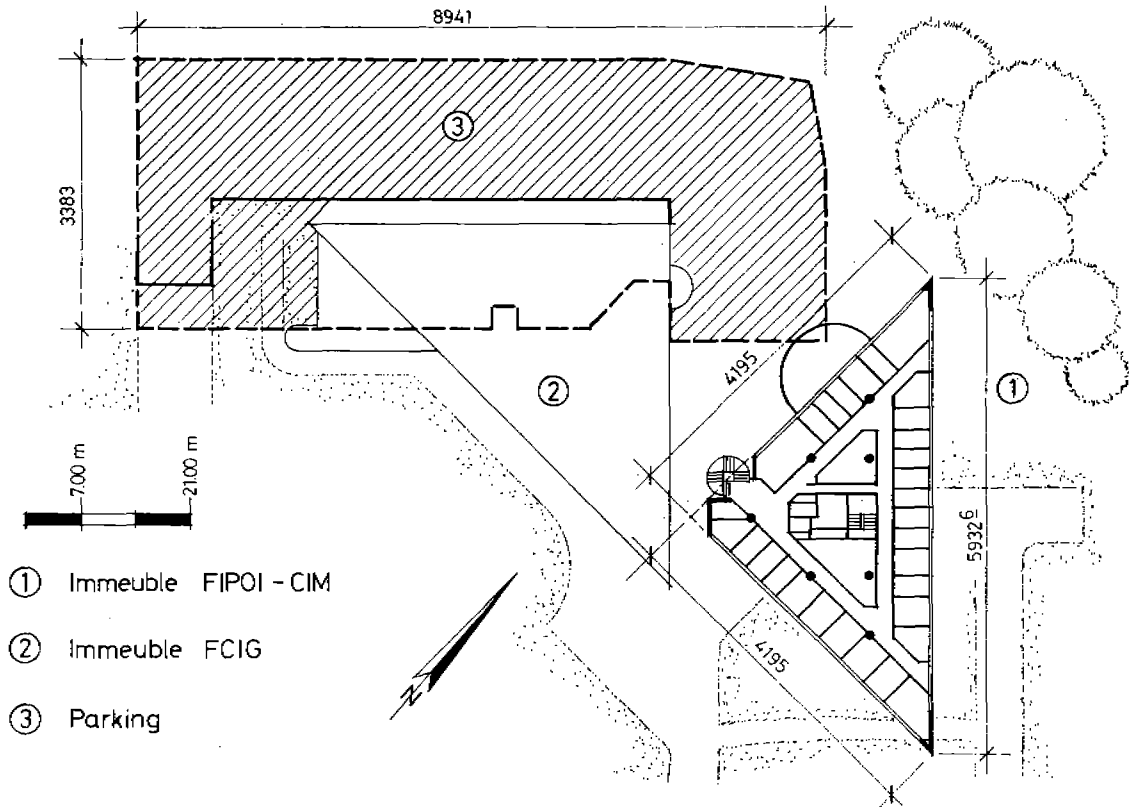
Plan horizontal du Centre administratif de Morillon (CAM)
