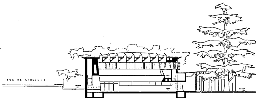
COUPE F-F
